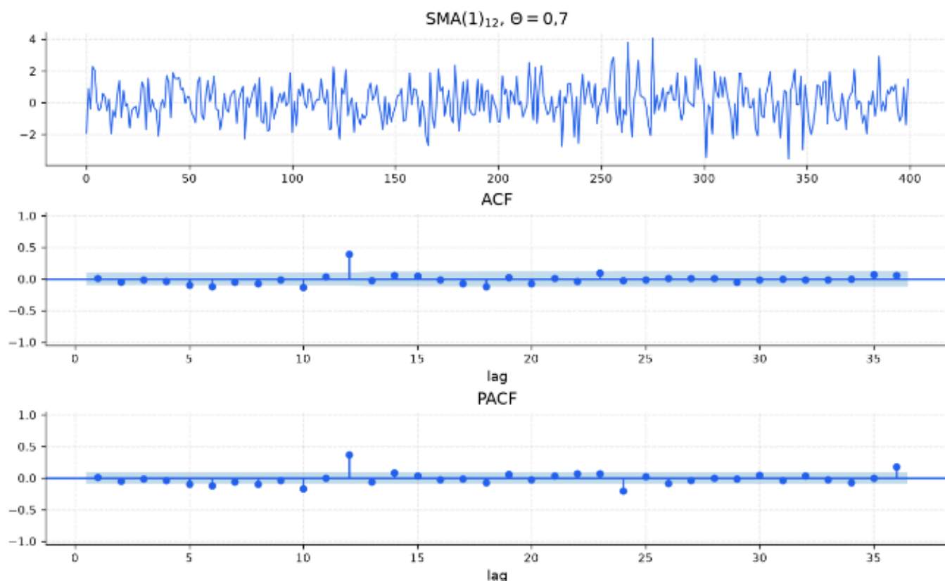
Figura 31: Identificação de ordens sazonais (P, Q) a partir da ACF e PACF
