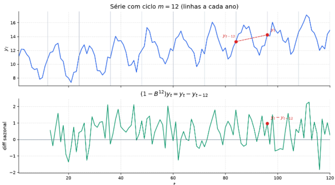
Figura 30: Série sem diferenciação sazonal e com diferenciação sazonal ( D=1 e m=12 )
